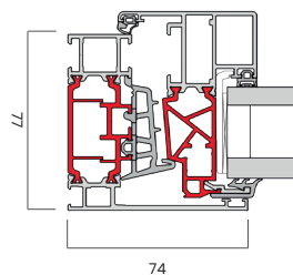
› C77K-CS SEZIONE LONGITUDINALE
