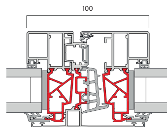
› C77K-CS NODO CENTRALE
